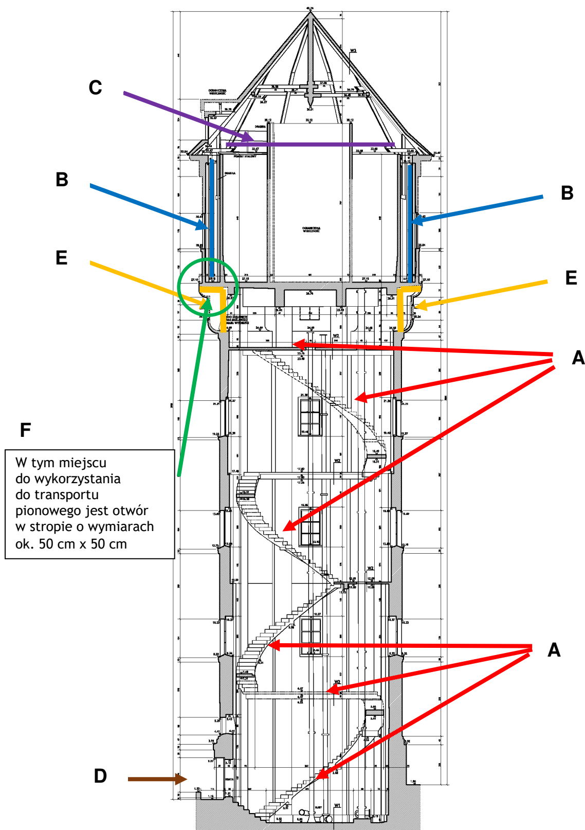
Rys. 1. Przekrój wieży przedstawiający:
